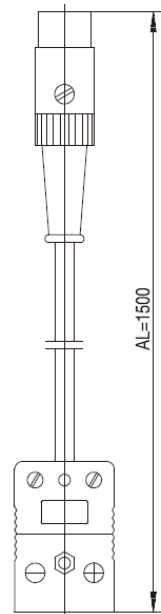
热电偶 (NiCr-Ni "K" 偶) 温度测量系统连接电缆
