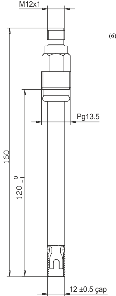
Tip 202922/30-... M12 konnektörlü dişli başlık
