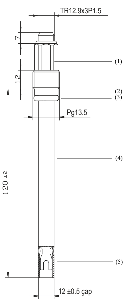
Tip 202922/30-... Pg13.5 dişli başlık
