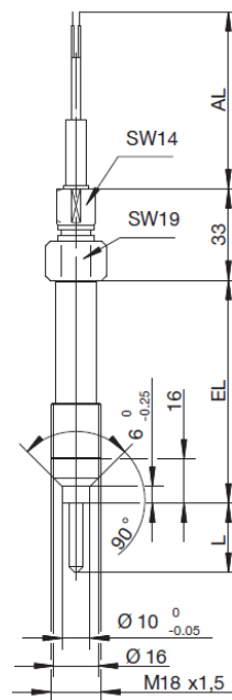
型号 902090/10 M18x1.5
