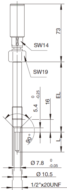
型号 902090/60... 1/2"x20UNF
