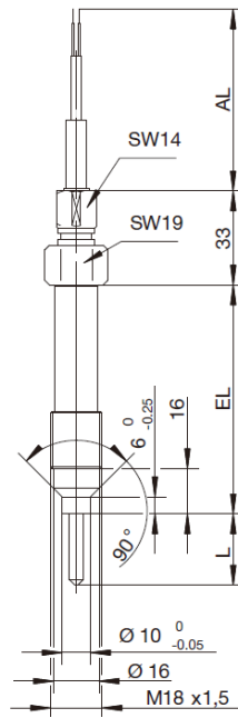
型号 902090/50 M18x1.5
