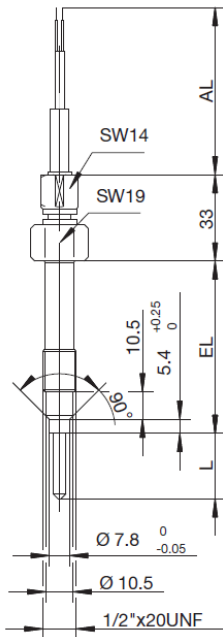
型号 902090/10... 1/2"x20UNF
