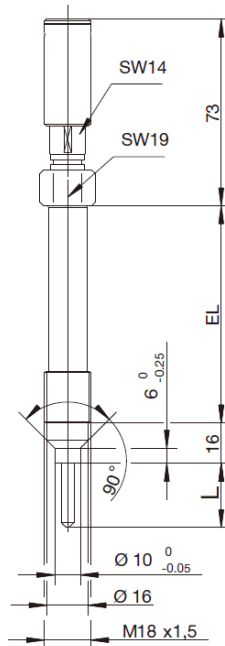
型号 902090/60 M18x1.5
