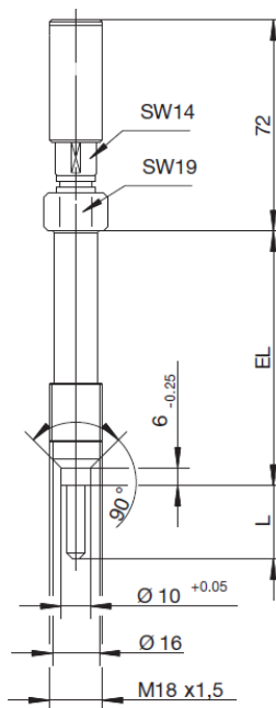
型号 902090/20 M18x1.5
