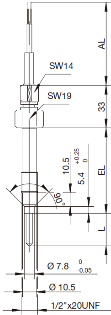
型号 902090/50... 1/2"x20UNF
